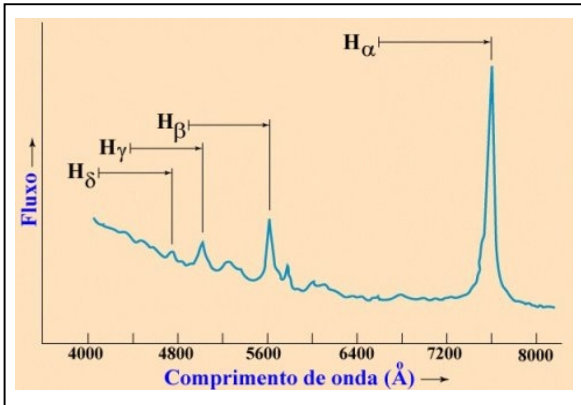
Figura 6.15 – Posição das linhas de emissão do H observadas em quasares típicos. As linhas horizontais em H_{\alpha} , \beta , \gamma , \delta representam a magnitude do deslocamento, em unidades de comprimento de onda.
