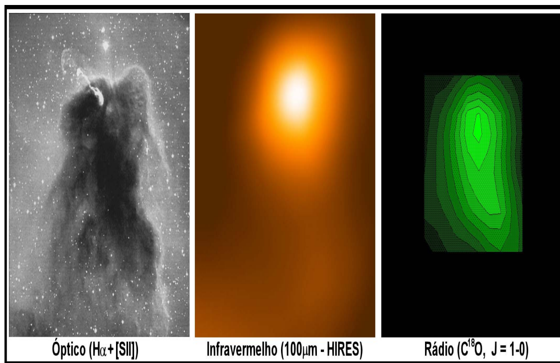
FIGURA 4 – Imagens óptica,, infravermelho e rádio do Glóbulo Cometário VG33. A imagem óptica é uma composição de imagens obtidas em \text{H}\alpha e \text{SII} (Reiputh, 1997) e a imagem radio é a emissão de \text{C}^{18}\text{O} (Hickel e Vilas-Boas, 2001)
