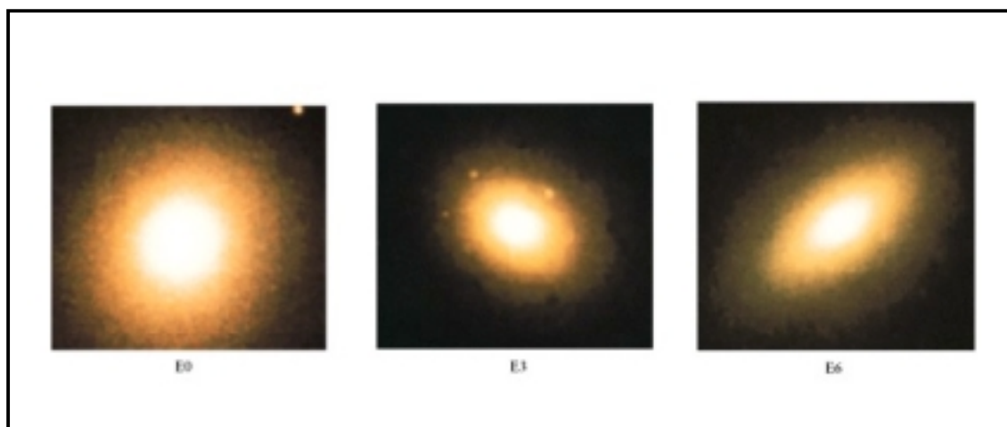
Figura 6.6 – Galáxia elíptica E0, E3 e E6. Note-se o gradual aumento de excentricidade da esquerda para a direita.
