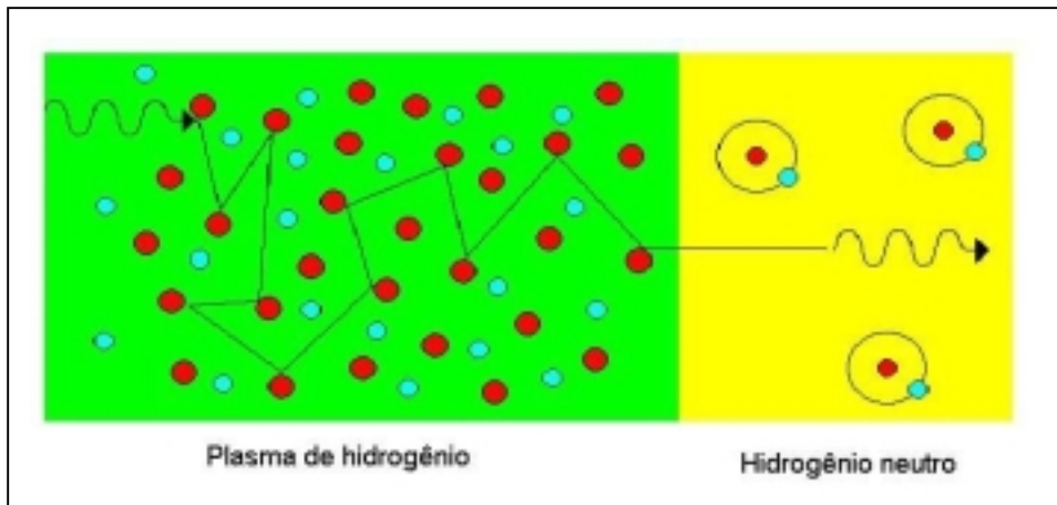
Figura 7.3 – O desacoplamento da matéria comum da radiação. Na figura à esquerda, o espalhamento Thomson obriga os fótons a percorrerem um caminho aleatório. Após a recombinação, os fótons podem ser propagar livremente pelo Universo.
