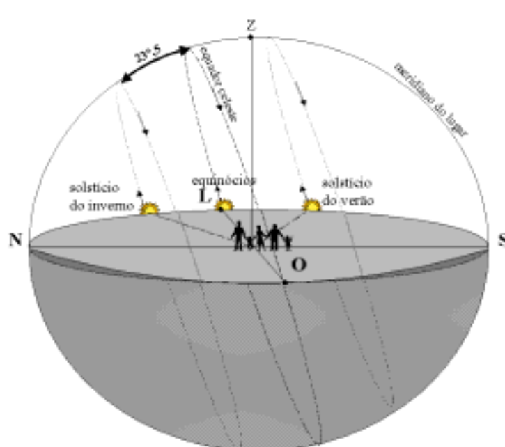
FIGURA 1.8 - VISÃO TOPOCÊNTRICA PARA O NASCER DO SOL NOS SOLSTÍCIOS E EQUINÓCIOS PARA UM LUGAR TROPICAL DO HEMISFÉRIO SUL DA TERRA.
