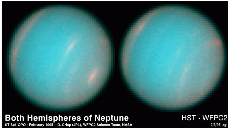
FIGURA 3.12 – IMAGENS DOS DOIS HEMISFÉRIOS DO PLANETA NETUNO OBTIDAS COM O HUBBLE SPACE TELESCOPE (STSCI).
