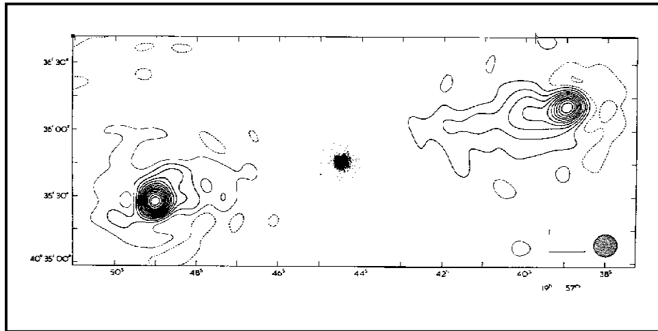
Figura 6.13 – Mapa em rádio de Cignus A, uma radiofonte clássica. A imagem central (na forma de uma pequena borboleta) representa a região emissora no óptico. As duas estruturas simétricas em relação ao centro são os chamados lobos emissores e emitem uma enorme quantidade de energia na faixa de rádio. O tamanho típico dessas estruturas em rádio é da ordem de alguns milhões de anos-luz.
