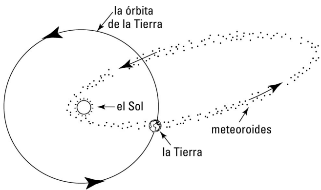
Figura 4-1: Cuando el camino de la Tierra cruza un
