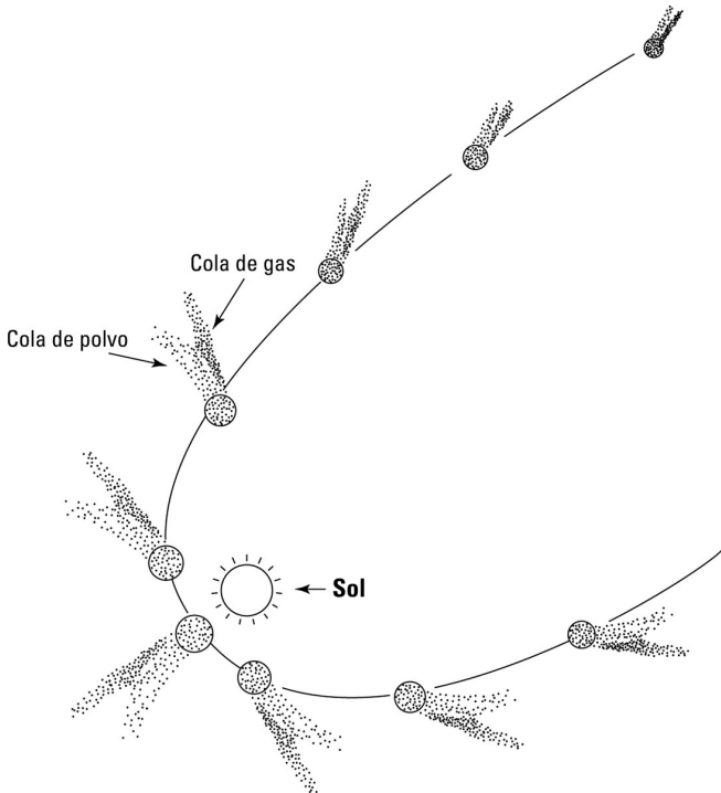
Figura 4-4: La cola de un cometa apunta en dirección
