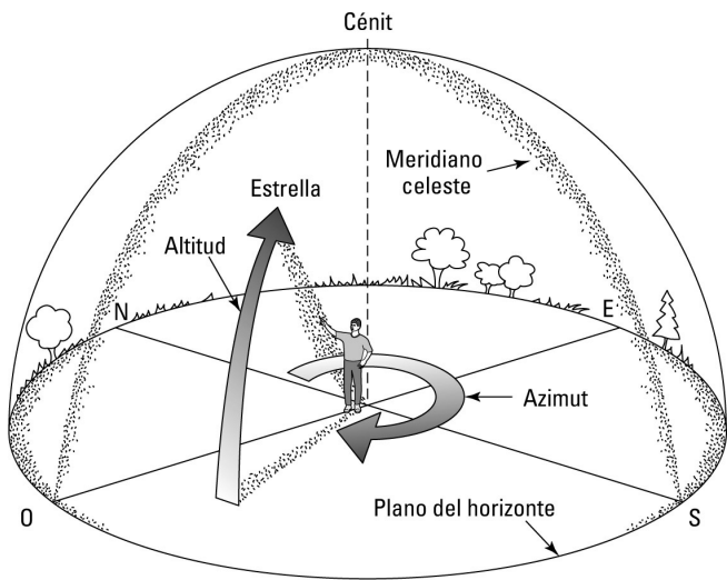
Posiciones en el cielo
