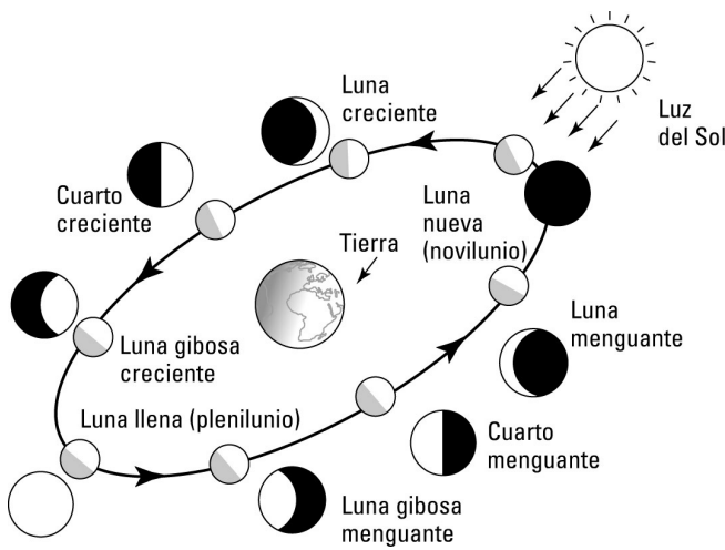
Figura 5-4: Las fases de la Luna. ¡Nos vemos en el otro lado!
