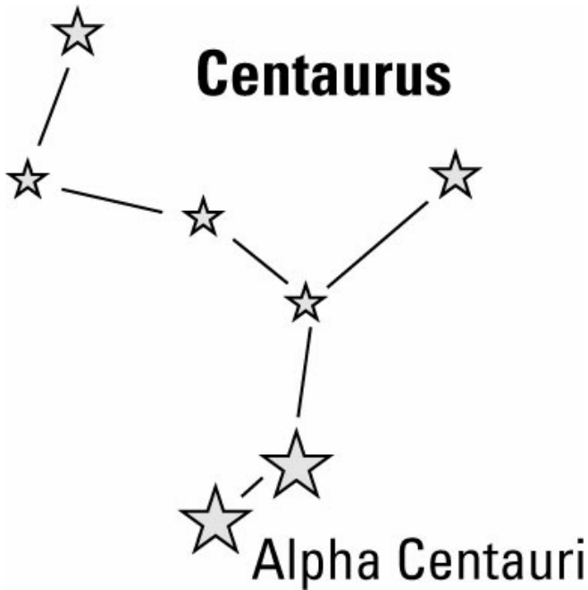
Figura 11-6: Alfa Centauri es un sistema de estrellas triple situado muy al sur en el cielo
